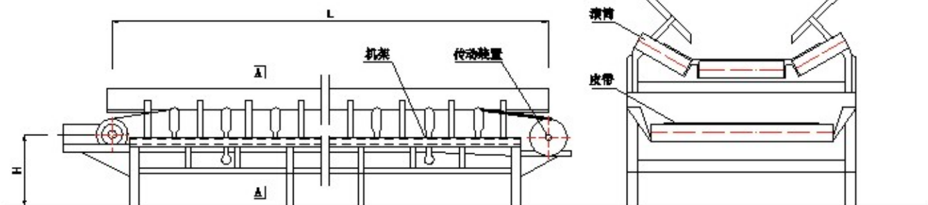
皮带式输送机技术选型示意图
