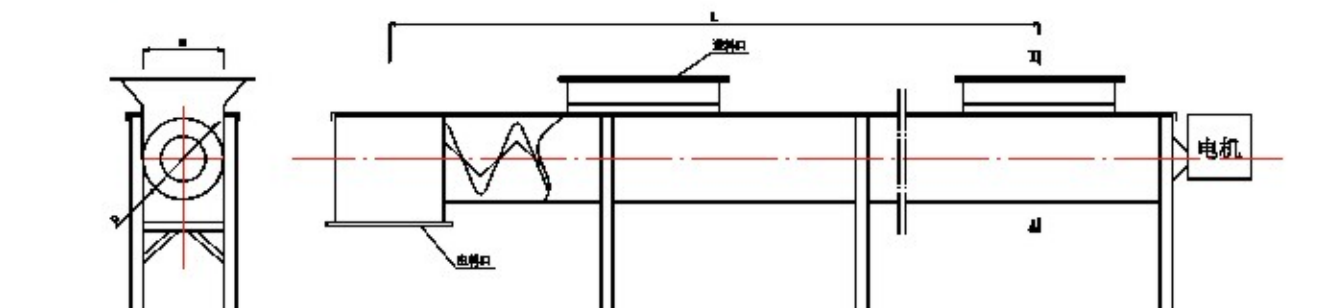
无轴螺旋输送机设计选型示意图
