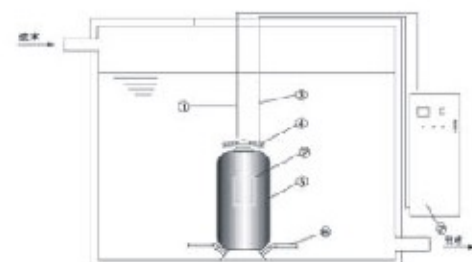
内置式水箱自洁消毒安装示意图
