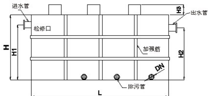
一体化污水处理设备示意图
